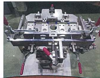
【電池】 燃料電池用 試作溶接治具
